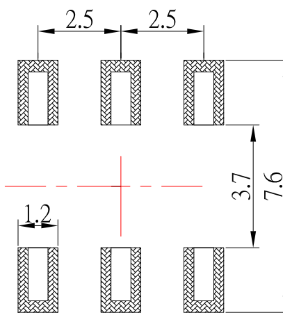
P.C.B LAND PATTERN
